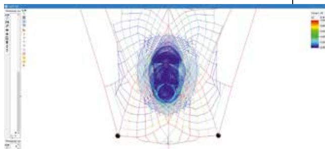
Рисунок 7. Вид по меридиану на разноглубинный трал Figure 7. Meridian view of a midwater trawl
