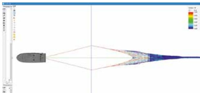
Рисунок 6. Вид сверху на разноглубинный трал Figure 6. Top view of a midwater trawl
