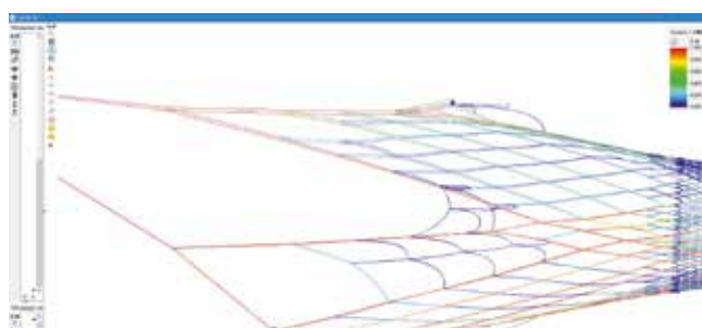
Рисунок 8. Натяжение в канатных связях (спектр) Figure 8. Tension in ropes (spectrum)
