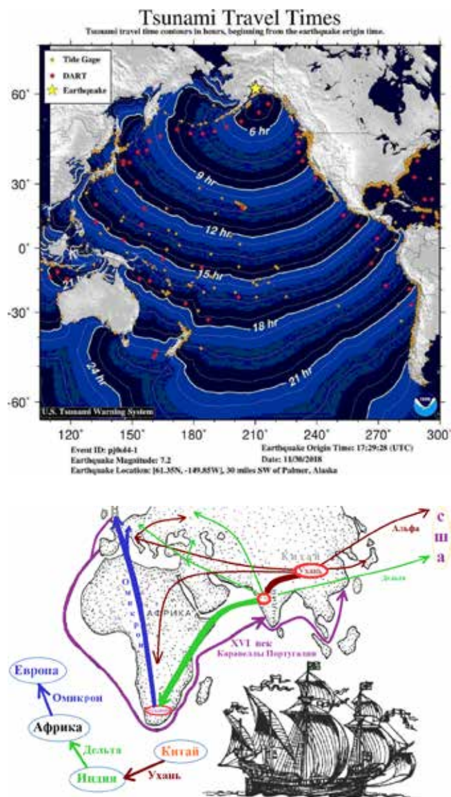
Рисунок 3. Сопряженность масштабов распространения океанологического цунами [12], путей португальских каравелл, сукцессии и пути распространения доминирующих штаммов КВ-19 [инет свободный доступ]
